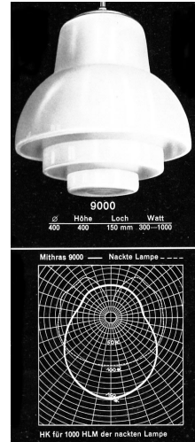
Mithras-Lampenschirm, Musterbuch 1938, darunter das Lichtintensitätsdiagramm
